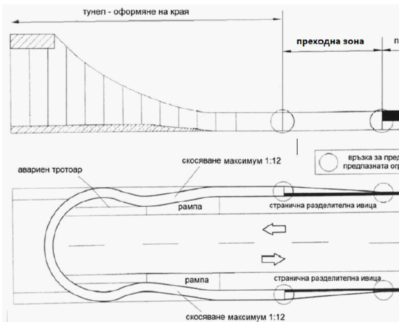
Фиг. 27. Оформяне на връзка между ограничителна система за пътища и начало на тунел
