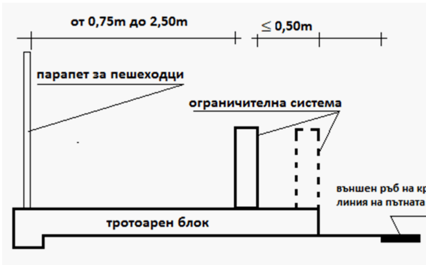
Фиг. 23. Място на ограничителна система върху тротоарен блок на съоръжение
