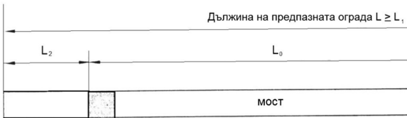
Случай б/: предпазна ограда върху мост с преходна зона
