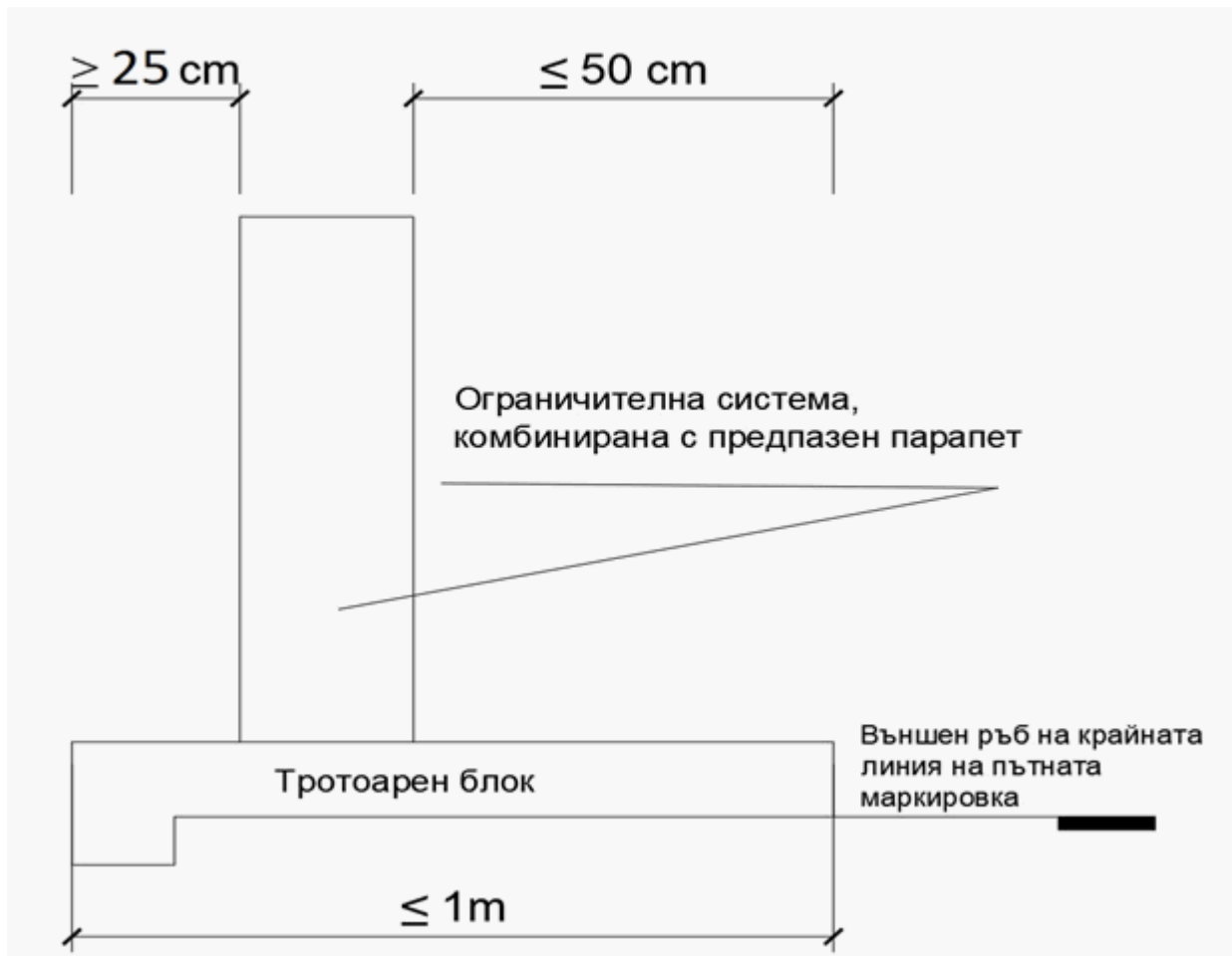
Фиг. 24. Място на ограничителна система, комбинирана с предпазен парапет върху тротоарен блок
